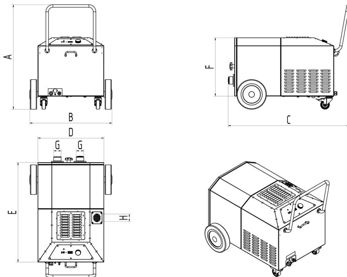
Fig. 17: Måleblad – produkt uten tilbehør
