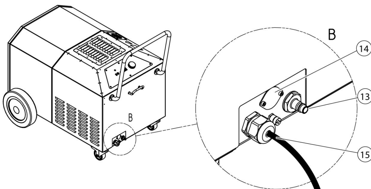
Fig. 2: Tilkoblinger
