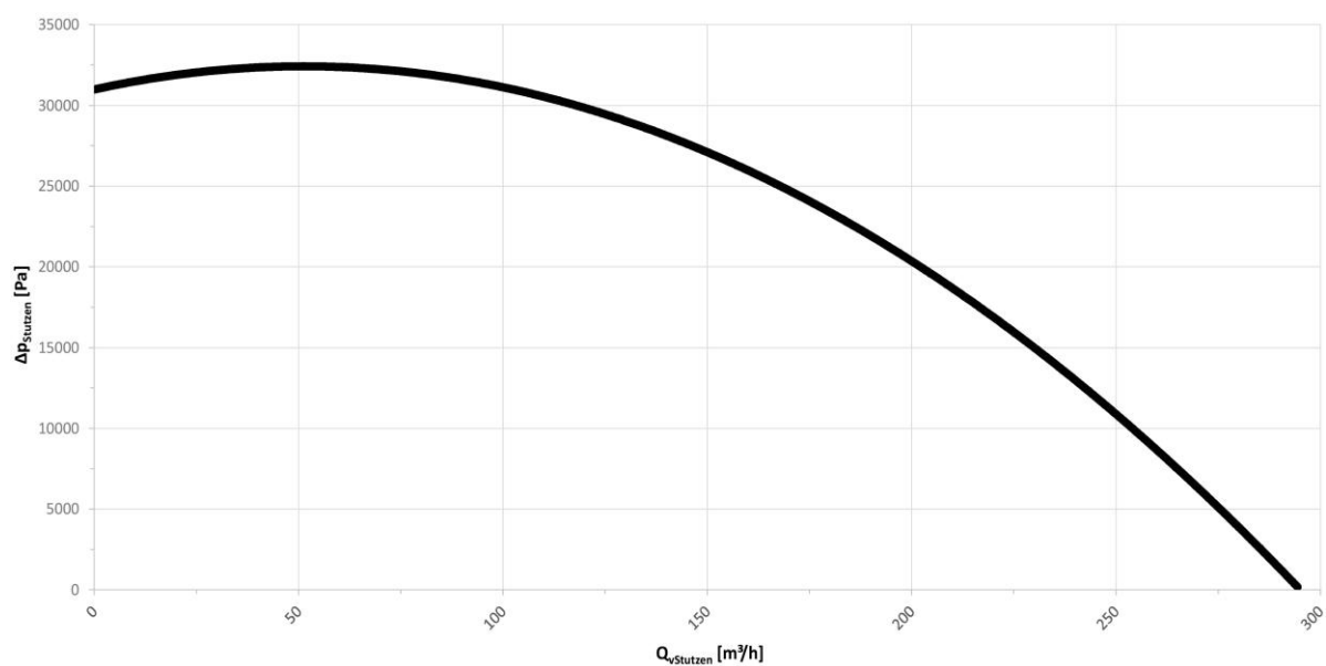
Fig. 16: Karakteristikk
