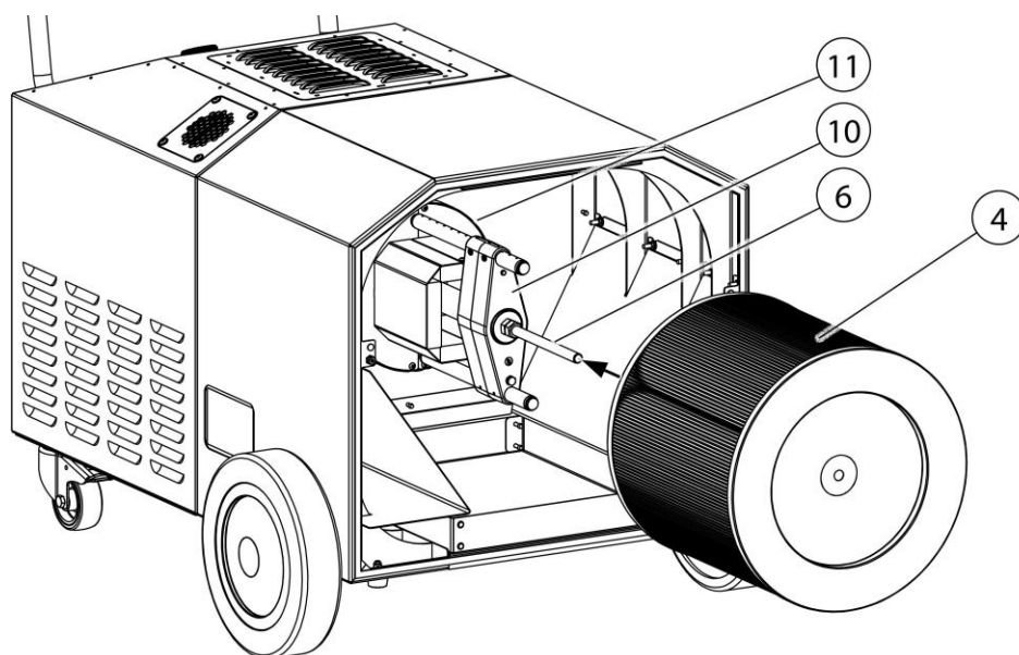
Fig. 12: Sette inn nytt hovedfilter
